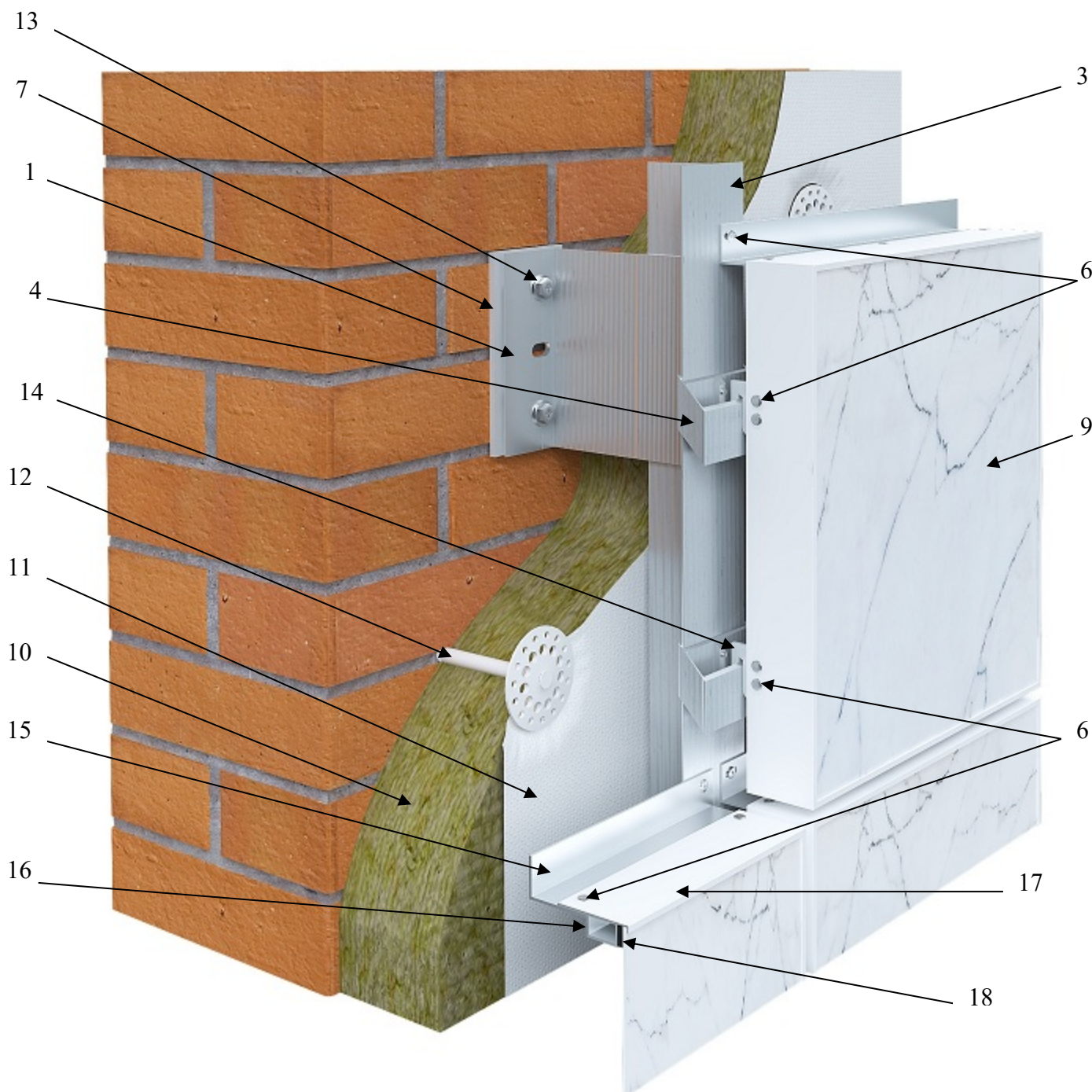
Рис. 6.1. Элементы фасадной системы MLK-v-300 со скрытым креплением кассетных панелей с лицевой поверхностью из керамогранита
