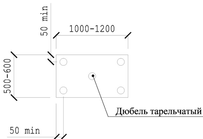
Схема крепления утеплителя (минераловатные плиты)
