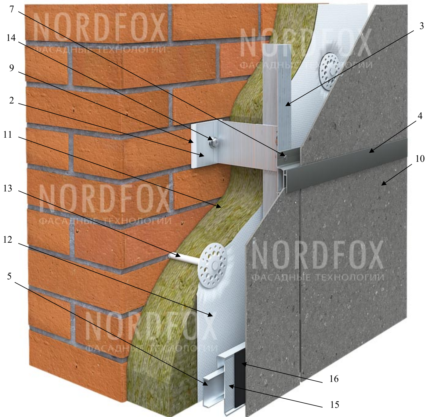
Рис. 6. Элементы фасадной системы MLK-v-300 с креплением облицовки с помощью горизонтальных планок, горизонтальных профилей и клипс
