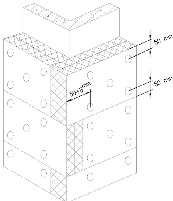
Схема крепления утеплителя на углу здания
