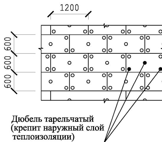
Схема установки внешнего слоя. Устанавливается с перевязкой горизонтальных и вертикальных швов минимум на 150 мм.
